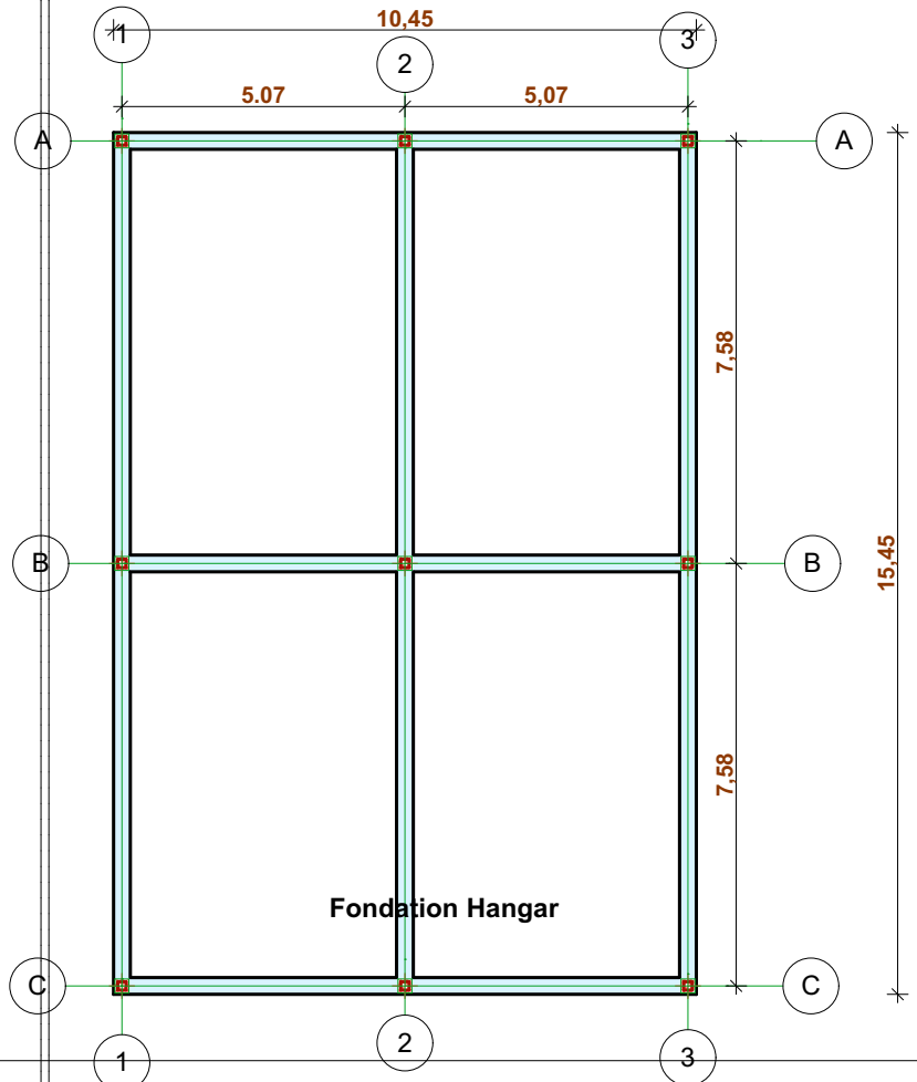
Plans de Fondation
