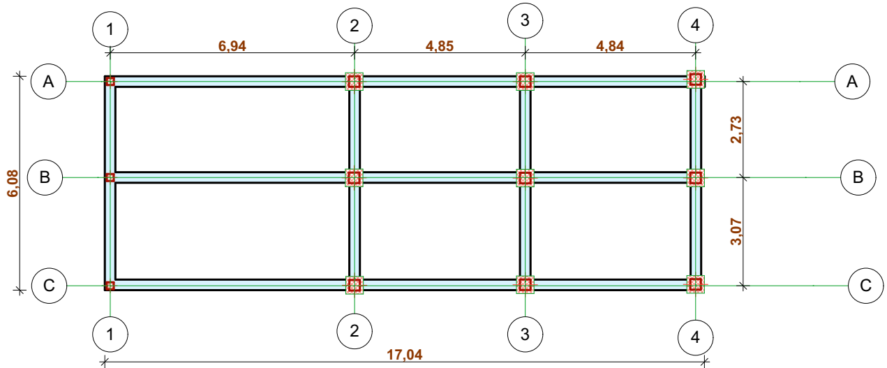
Plan de Fondation: Magasin et Bloc Administratif
