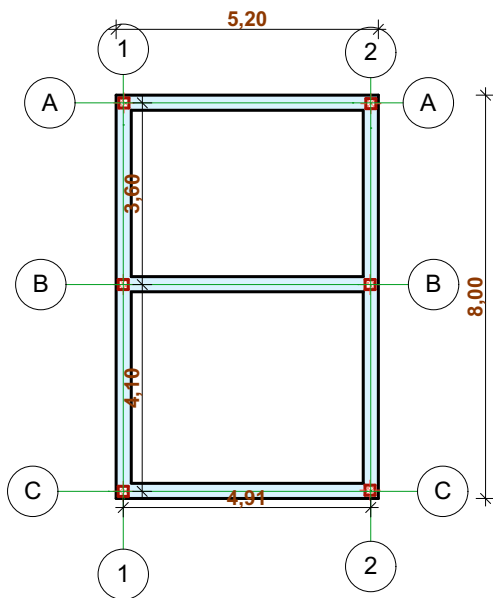
Fondation Cuisine restauration
